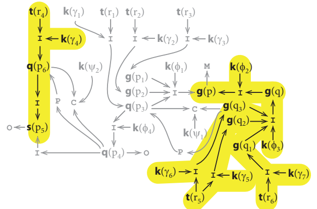
(d) Candidate solution r-net B is highlighted.
